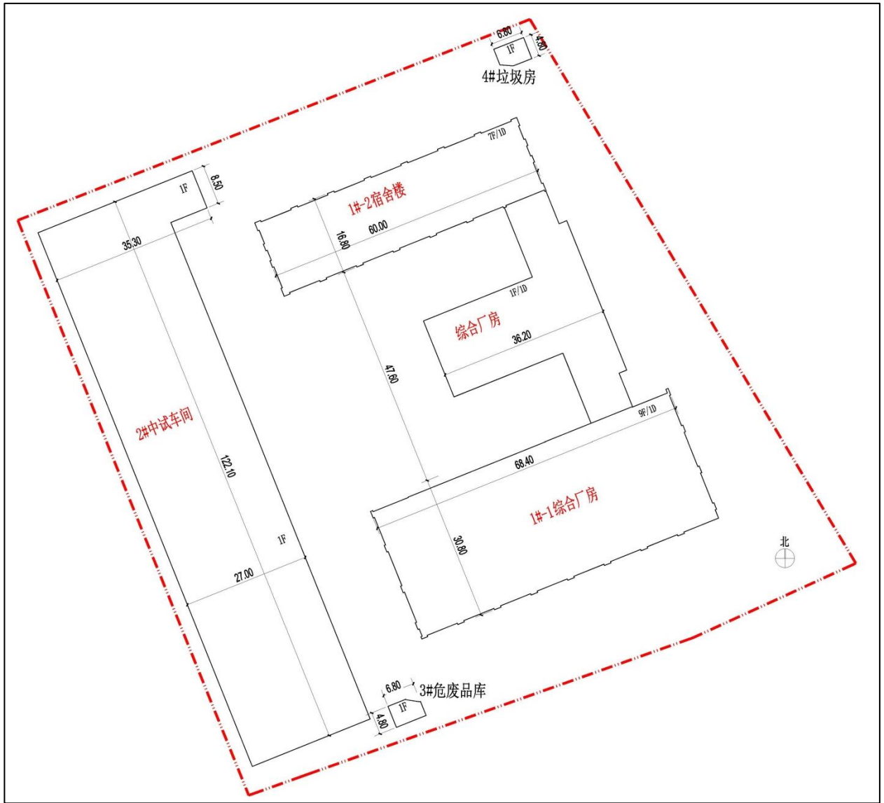
图 1.5-1 建筑总平面示意图
